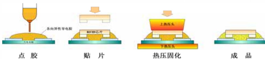
一种采用各向异性导电胶互连的RFID标签制造过程示意图
