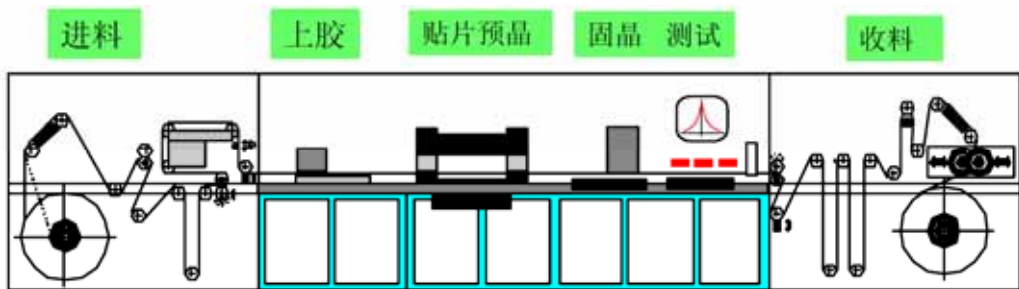
“卷对卷” (Roll to Roll) 的大规模电子标签生产装备
