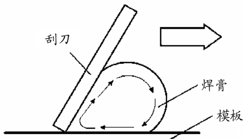
环形模板结构的焊膏可印刷性测试仪
