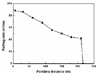
焊膏印刷距离与滚动速度的关系
