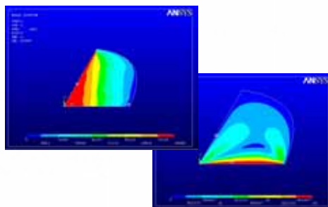
印刷过程中焊膏滚动现象的模拟
