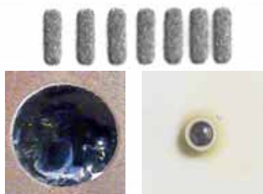
焊膏的热塌、收球与铜板润湿测试
